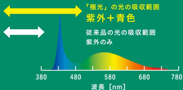
白色 LED の分光分布
